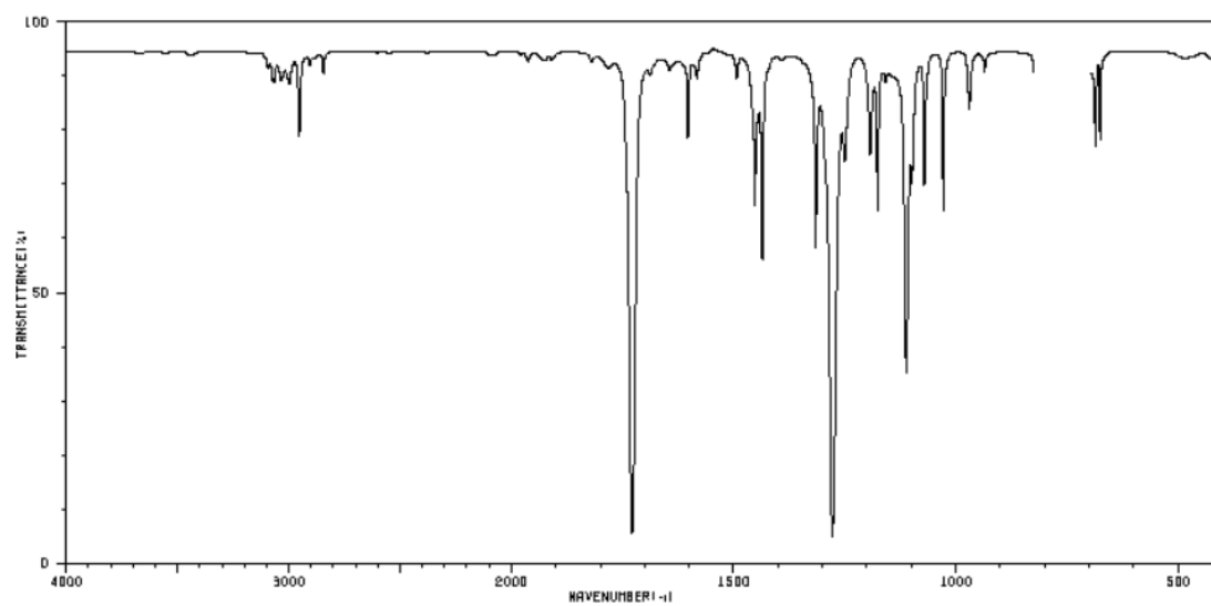
IR-A11 C_8H_6N_2O
