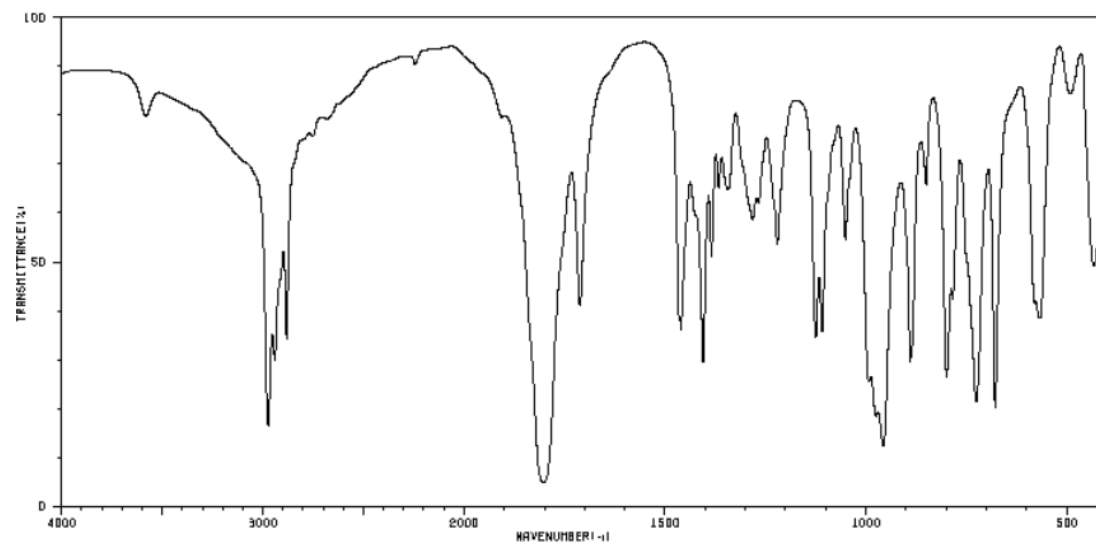
IR-A9 C 4 H 7 OCI
