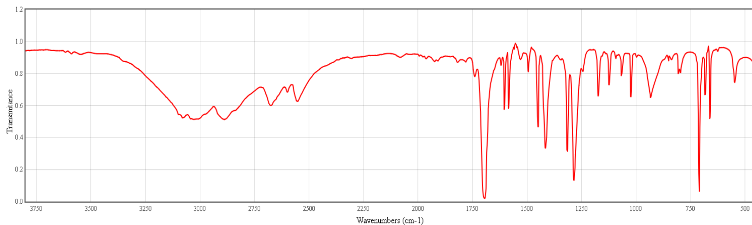
IR-A3 C 7 H 7 NO
