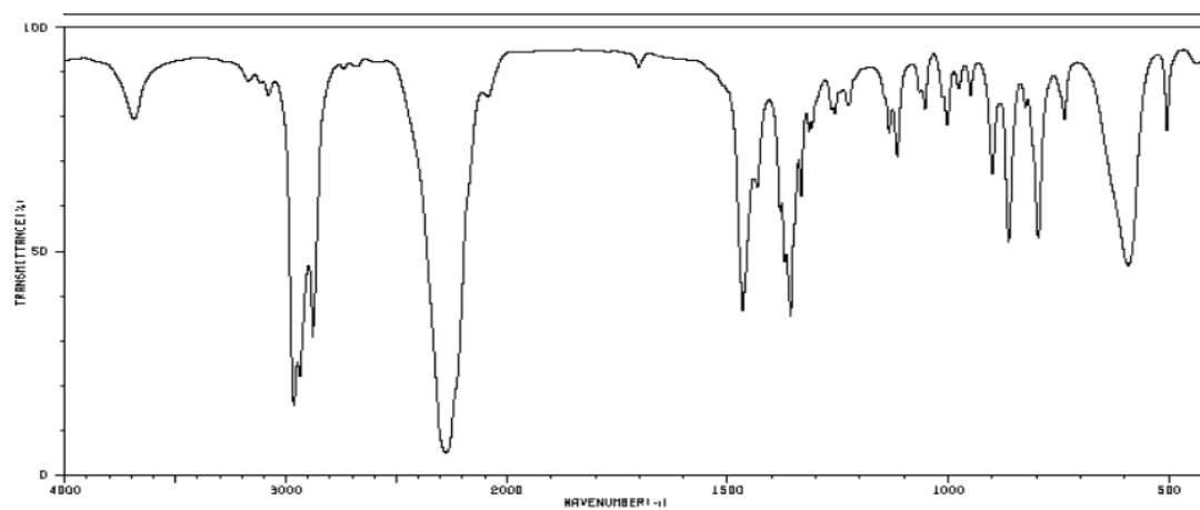
IR-A12 C_5H_9NO
