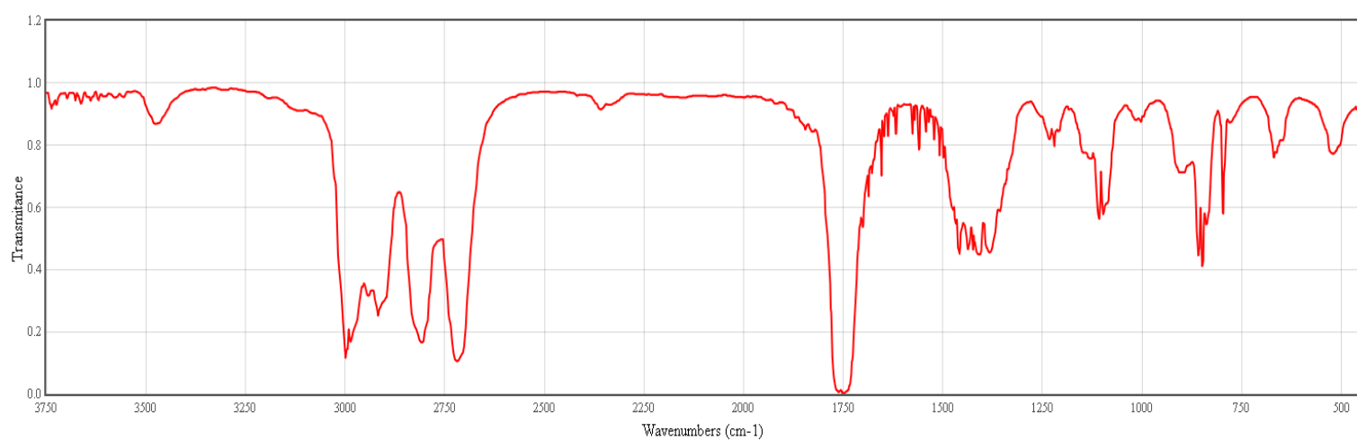
IR-A4 C 3 H 6 O
