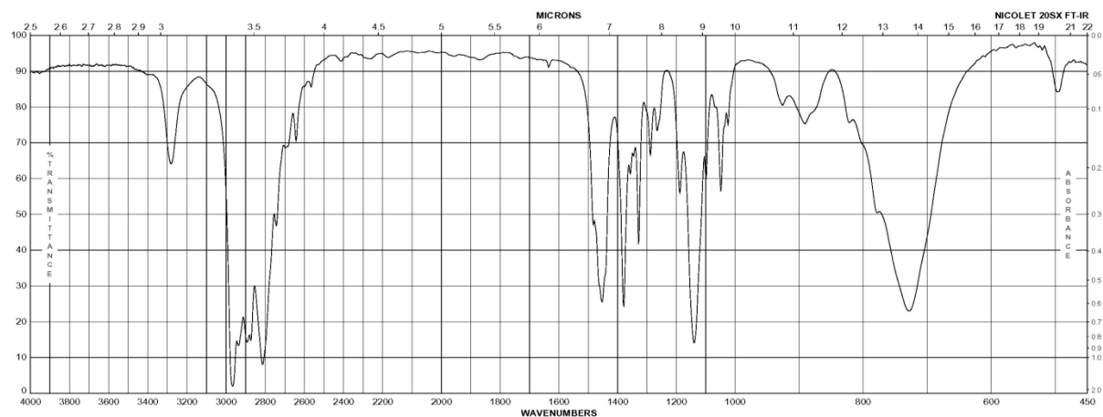
IR-A8 C 5 H 10 O
