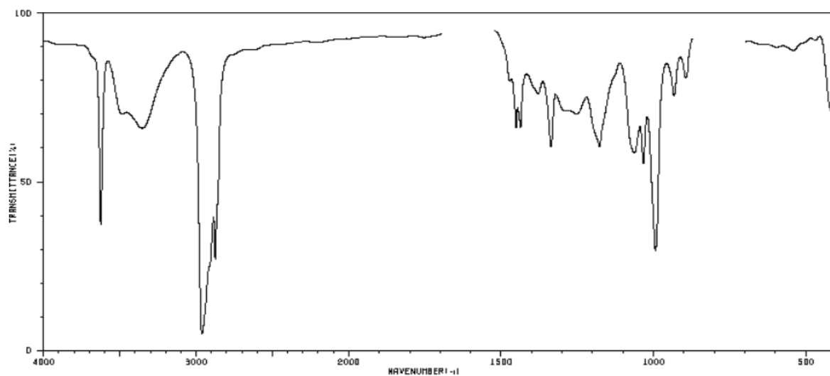
IR-A9 C 4 H 7 OCI
