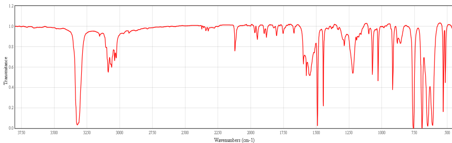
IR-A2 C 7 H 6 O 2
