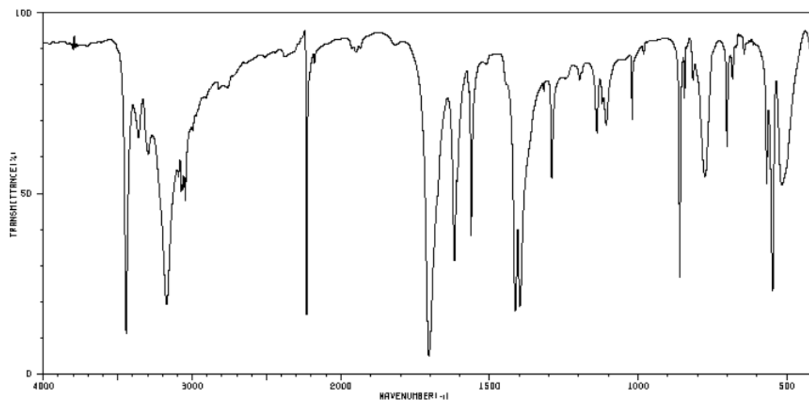
IR-A12 C_5H_9NO
