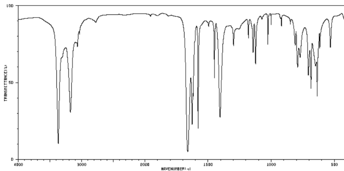
IR-A3 C 7 H 7 NO
